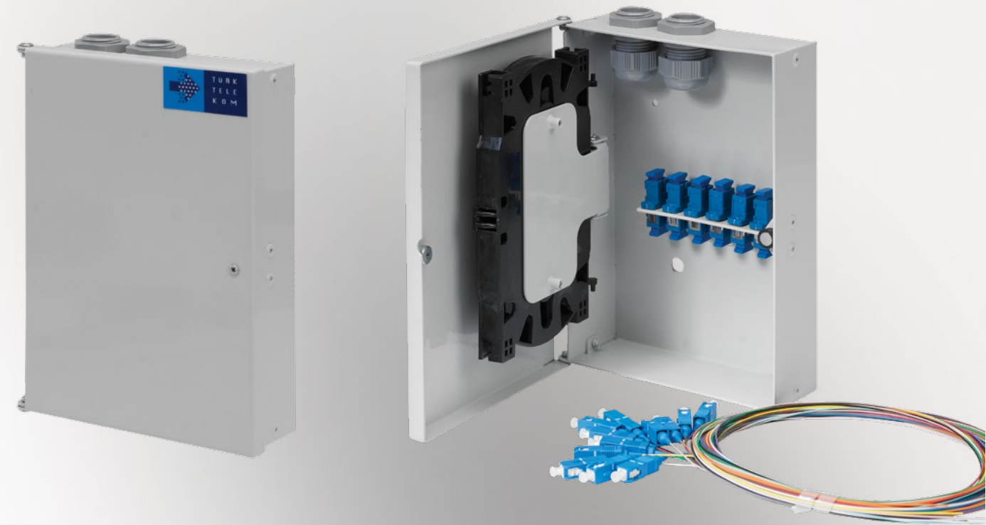
6 PORT ODF BOX
